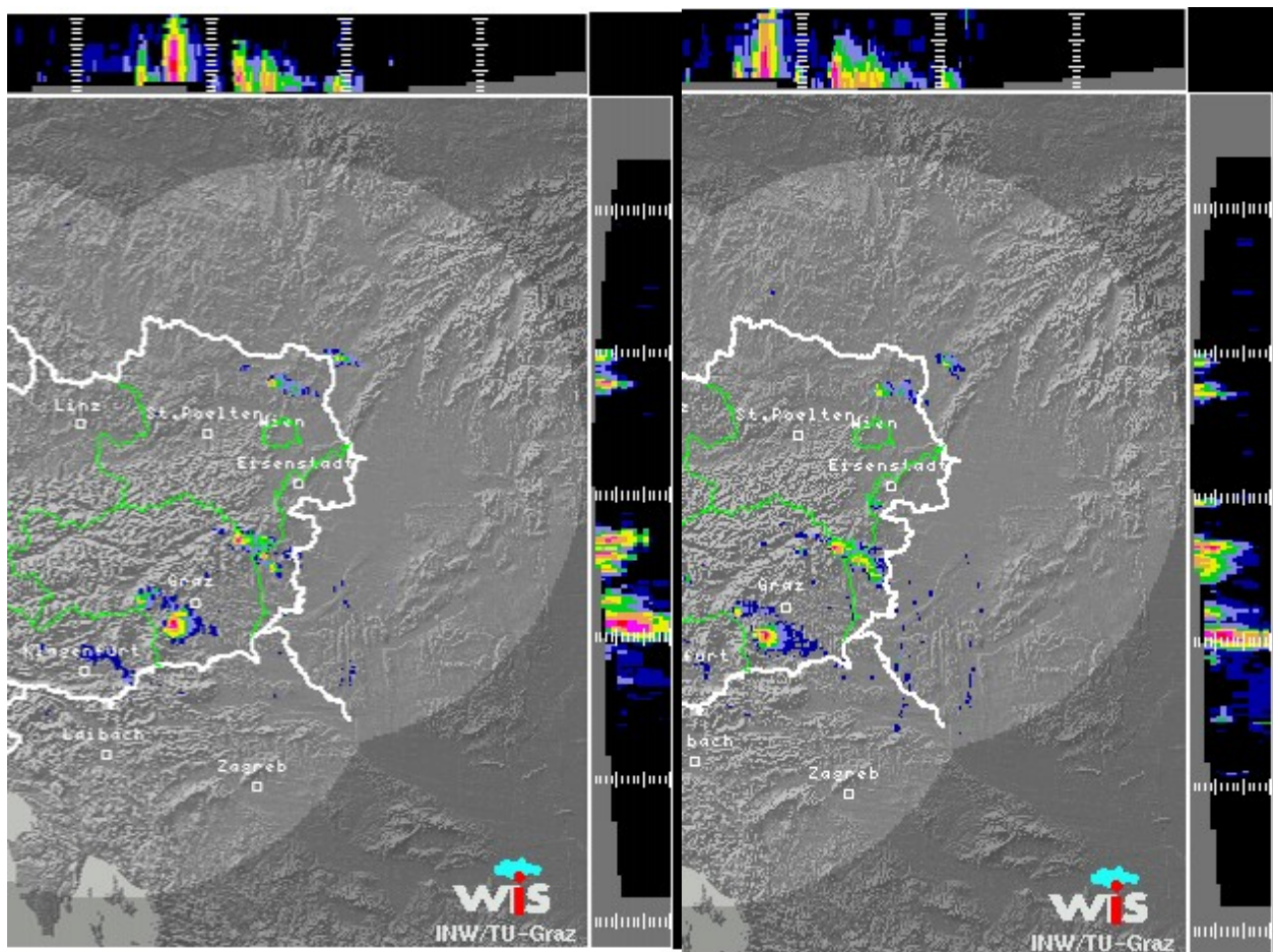
Radarbild 20080621 16:05
